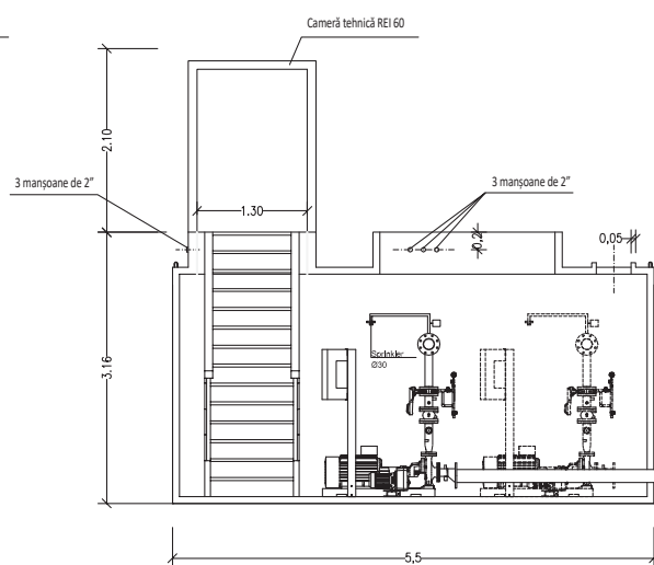
SECȚIUNE LONGITUDINALĂ A-A
