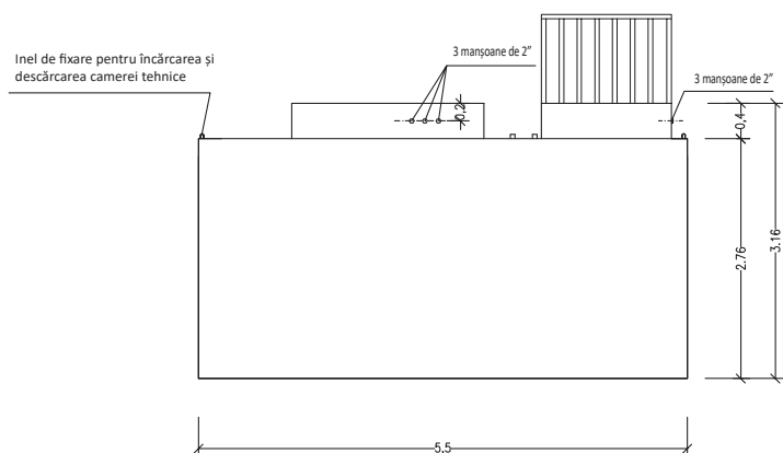
VEDERE LATERALĂ - 3
