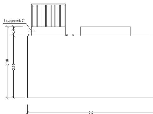
VEDERE LATERALĂ - 1
