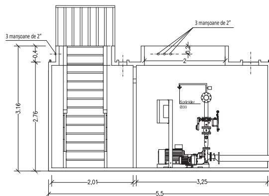
SECȚIUNE LONGITUDINALĂ A-A
