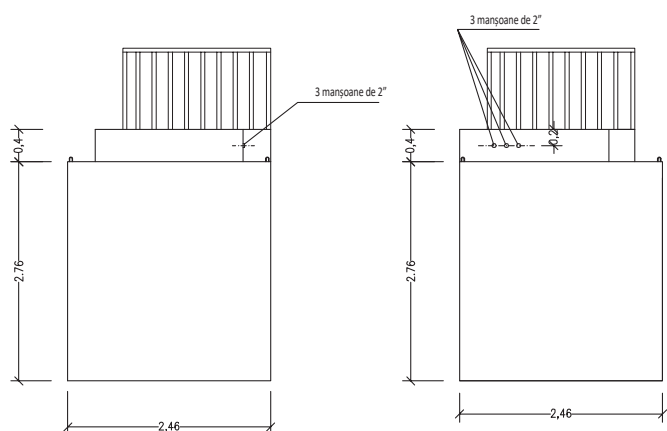
VEDERE LATERALĂ - VEDERE 4
