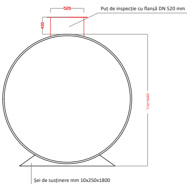
SECȚIUNE A-A
