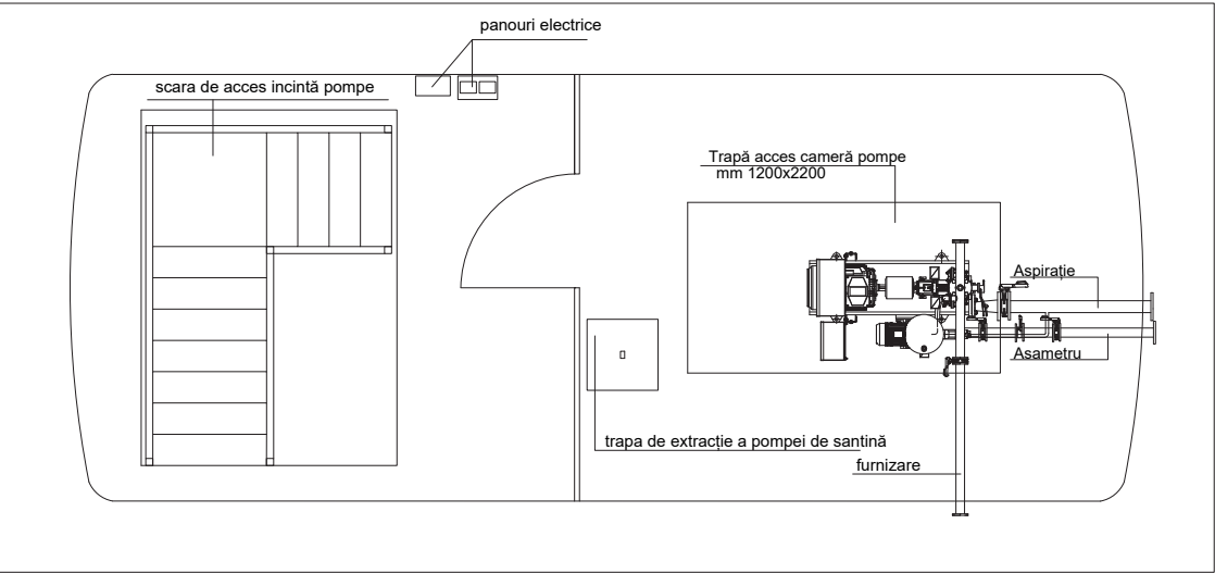
PLANUL CAMEREI TEHNICE
