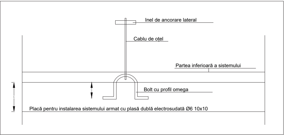
DETALIU ATAȘĂRII TIRANTELOR
